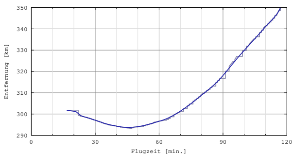
Abb. 5: Entfernung zwischen Ballon und dem Beobachtungsstandort - Quelle: Sven (DG1SVE)
