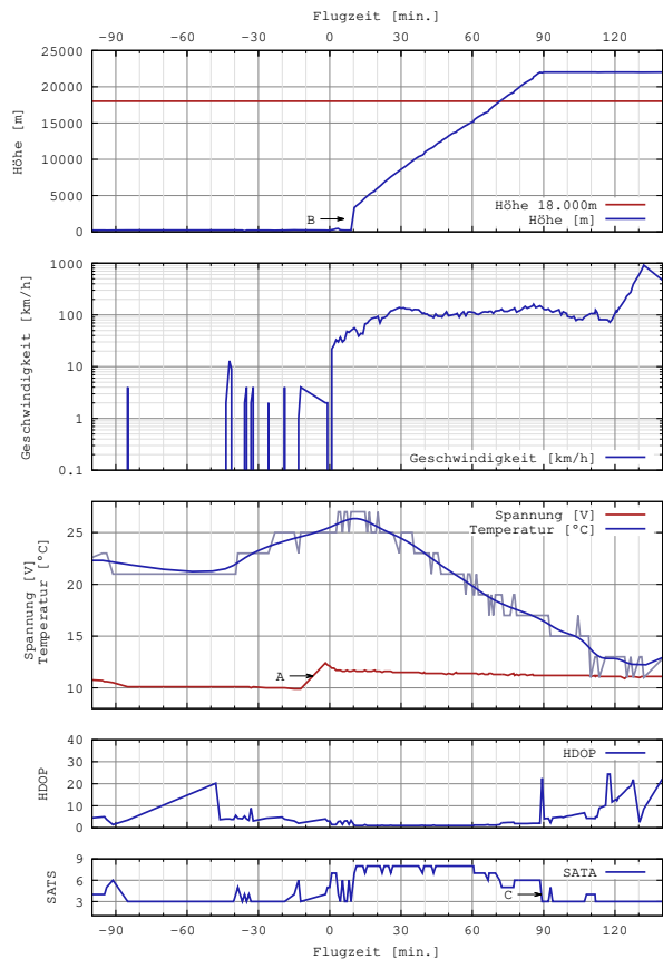
Abb. 3: Telemetriedaten - Quelle: Sven (DG1SVE)
