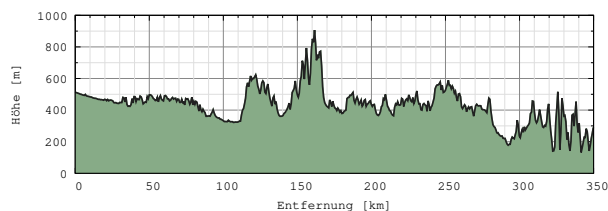
Abb. 7: Höhenprofil zwischen Ballon und DG1SVE, letzter direkter Kontakt - Quelle: Sven (DG1SVE)
